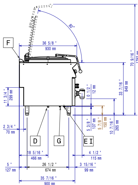
Zij aanzicht
