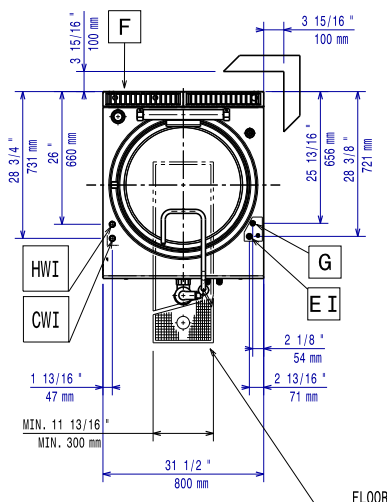
Boven aanzicht
